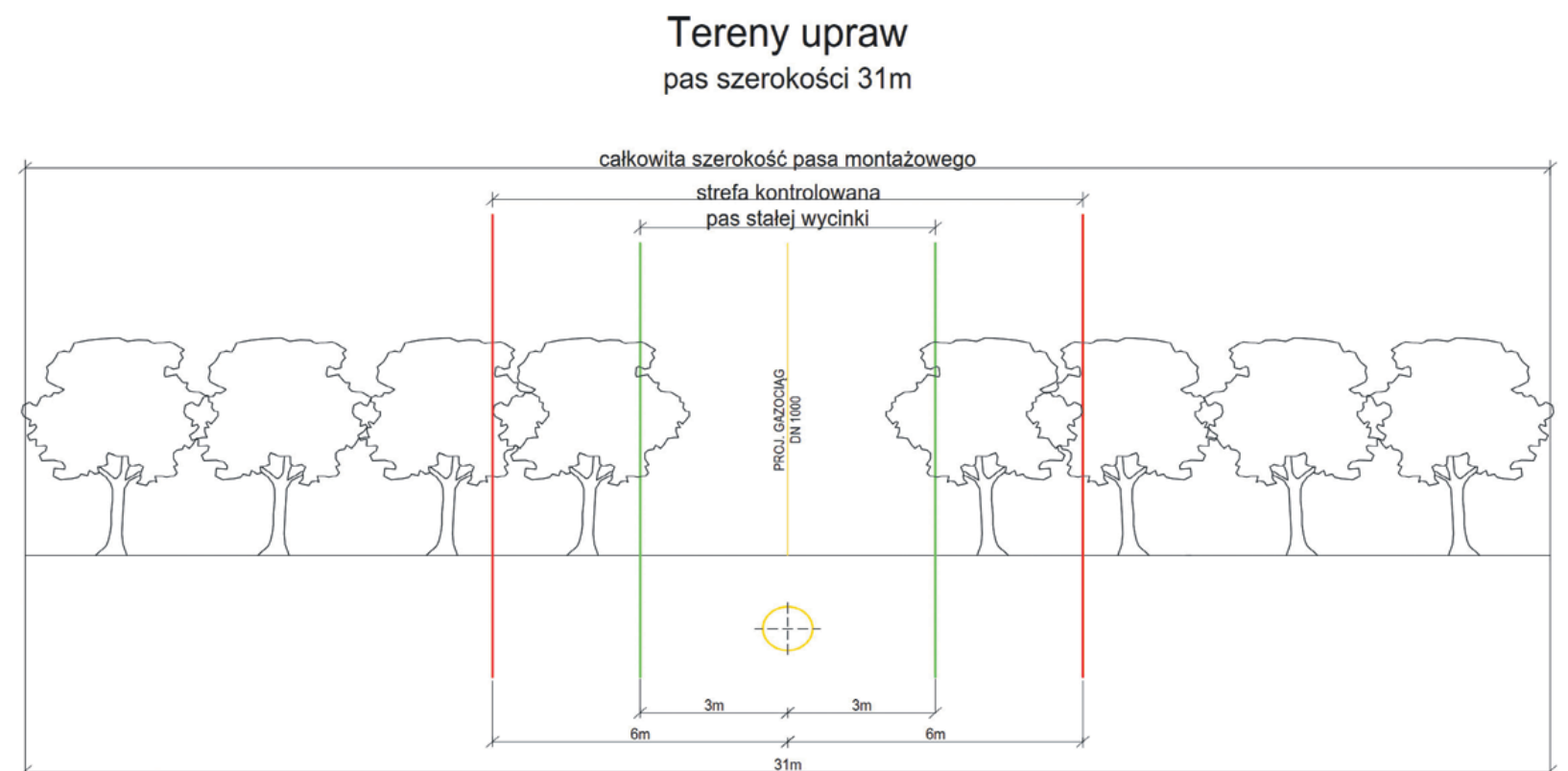
Rys. nr 1. Rysunek strefy kontrolowanej gazociągu.
